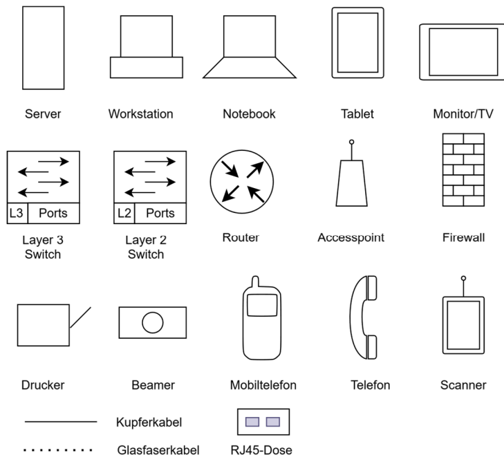
Abbildung 2: Symbole Netzwerkentwurf
